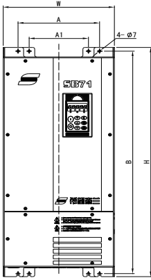
SB71G15-SB71G30 机型外形图
