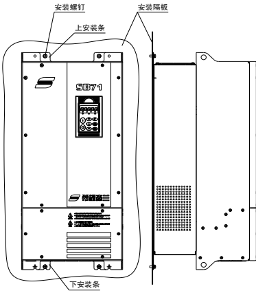
SB71G15-SB71G30 安装方式一
