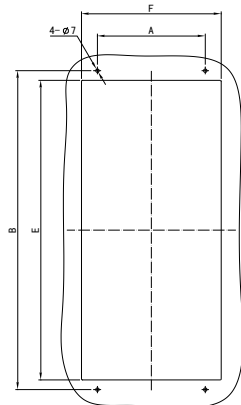
SB71G15-SB71G30 安装方式二开孔图
