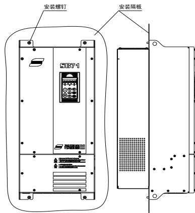
SB71G15-SB71G30 安装方式二
