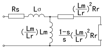
T-I型等效电路
