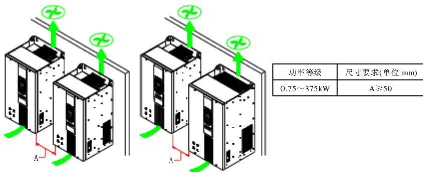
图 3-3 Hope590PM0.75T4~Hope590PM375T4 多台机器并排安装
