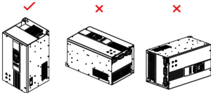
图 3-5 安装方向示意图
