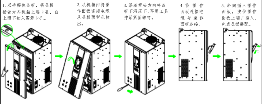
图 3-12 Hope590PM45T4~Hope590PM375T4 机型盖板拆卸与安装步骤
