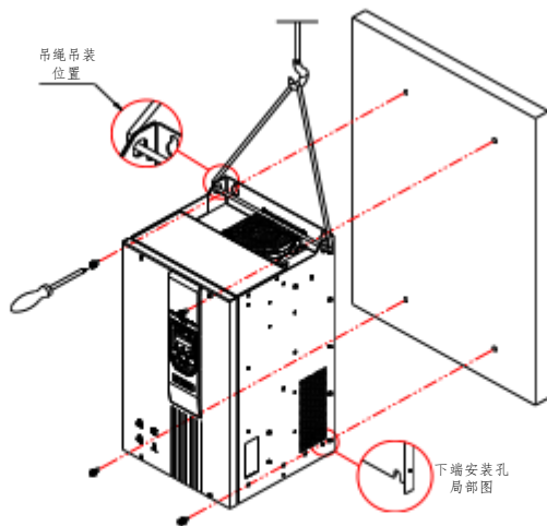
图 3-7 Hope590PM45T4~Hope590PM375T4 机型壁挂式安装
