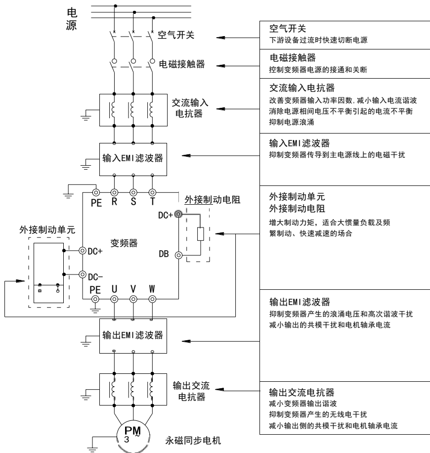
图3-13 Hope590PM系列变频系统连接示意图
