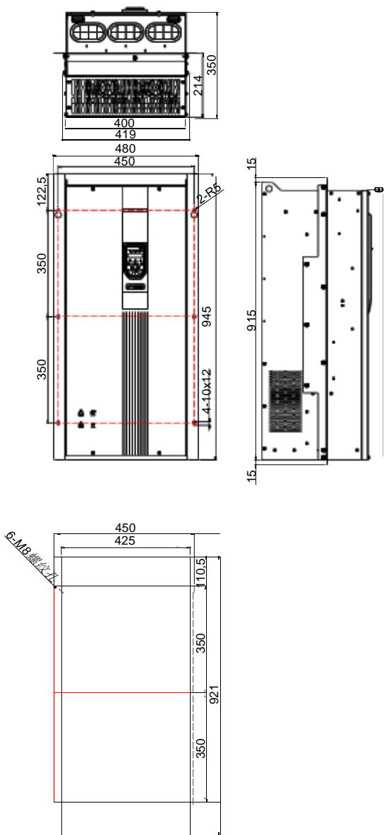
H590-A-6 安装挂条及开孔尺寸示意图
