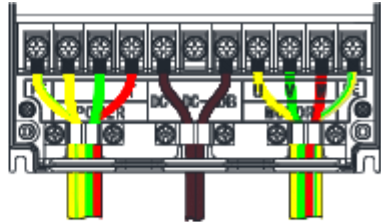
主回路端子整体接线效果图
