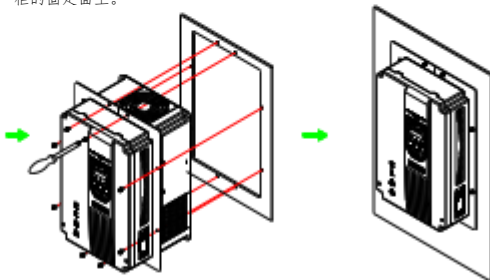
图 3-8 Hope590PM11T4~Hope590PM37T4 机型嵌入式安装
