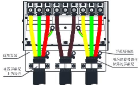
主回路端子整体接线效果图
