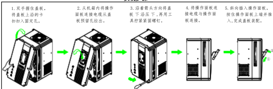
图 3-11 Hope590PM11T4~Hope590PM37T4 机型盖板拆卸与安装步骤
