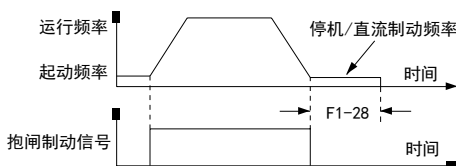
抱闸延迟时序图
