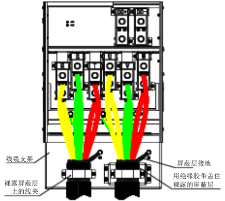
主回路端子整体接线效果图
