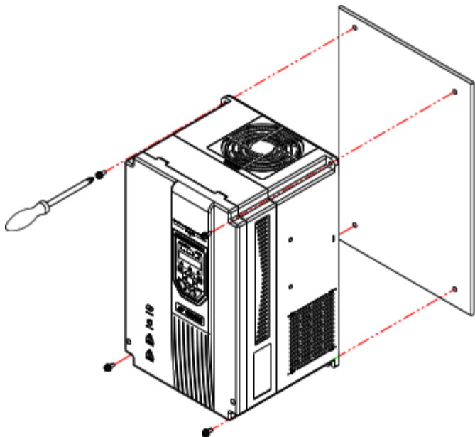
图 3-6 Hope590PM0.75T4~Hope590PM375T4 机型壁挂式安装
