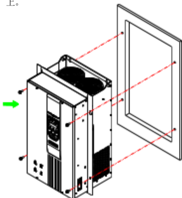
图 3-9 Hope590PM45T4~Hope590PM375T4 机型嵌入式安装
