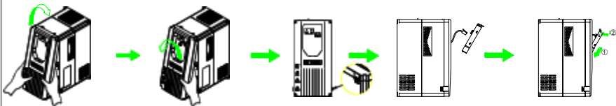
图 3-10 Hope590PM0.75T4~Hope590PM7.5T4 机型盖板拆卸与安装步骤
