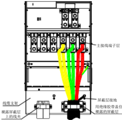
主回路端子输出端接线效果图
